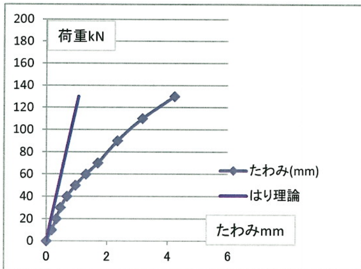
道路照明 鋼管柱 φ165.2の荷重とたわみ
