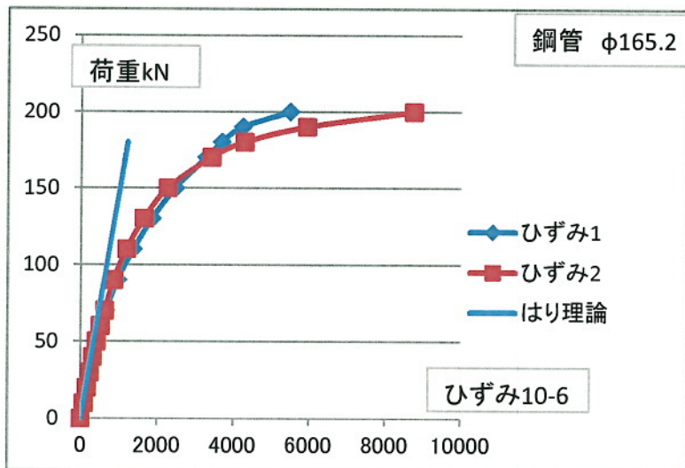
道路照明 鋼管柱 φ165.2の荷重とひずみ
