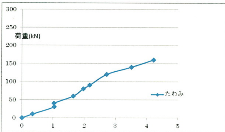
補強鋼管R1の荷重とたわみ
