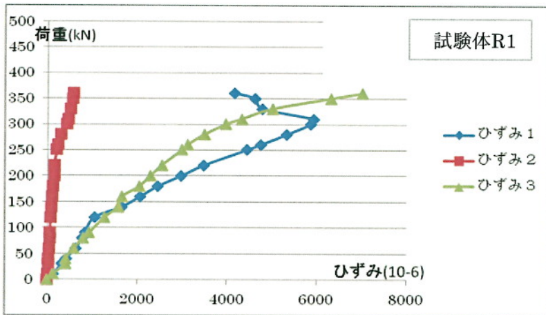
補強鋼管R1の荷重とひずみ
